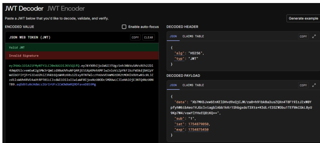
Gambar 4.36 Proses Decode Token JWT pada Website Jwt.io
